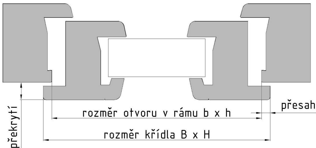
Obrázek 1 – Překrytí profilu křídla vůči profilu rámu
