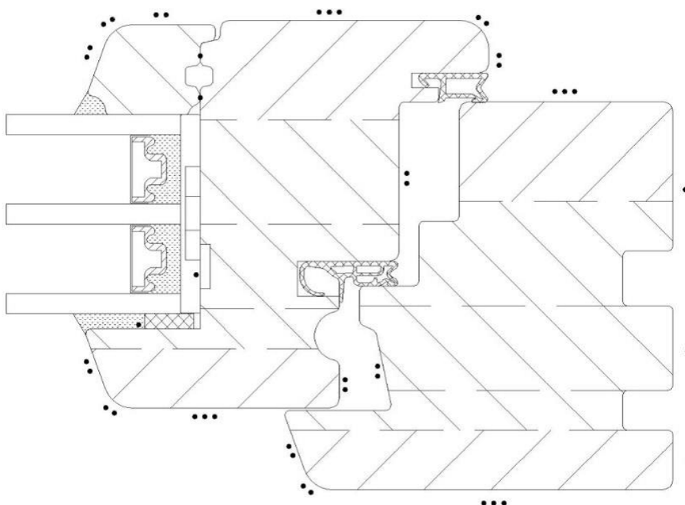
Obrázek 3 – Specifikace posuzovaných ploch dřevěného profilu
