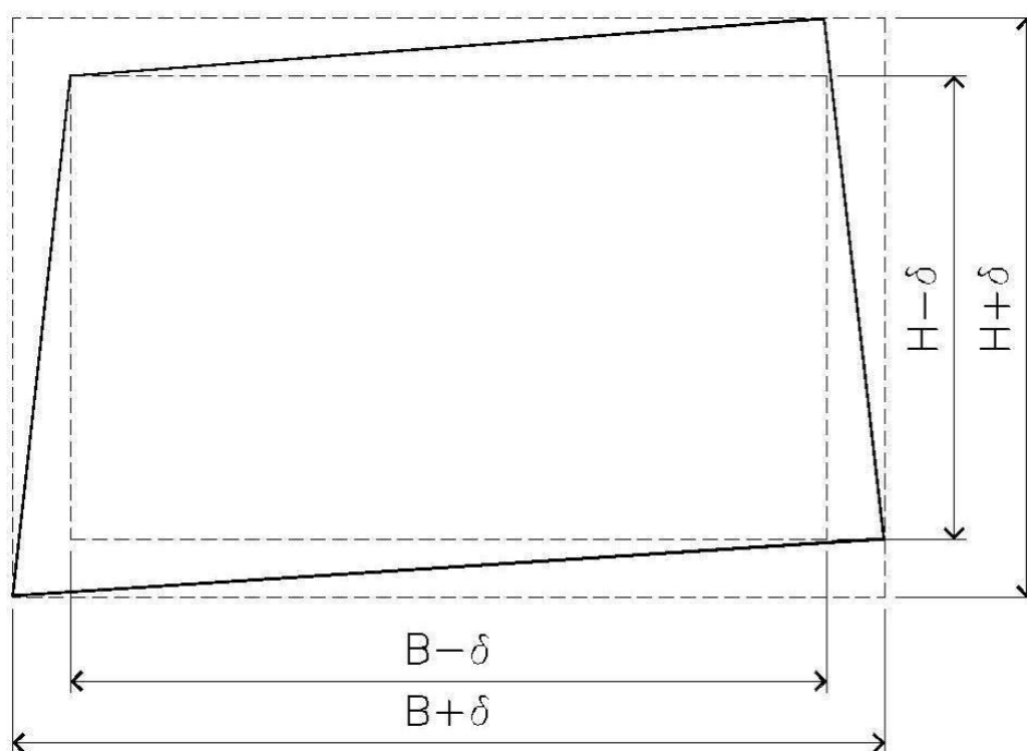
Obrázek 2 – Odchylky tvaru
